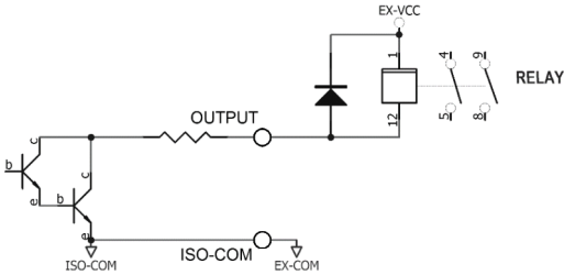
图9-2-6-1 控制继电器
