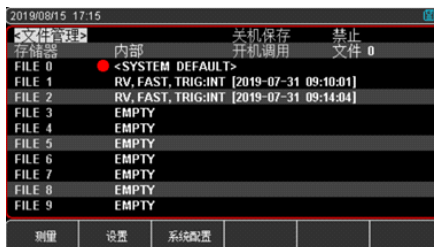
图 5-2 <文件管理>页
