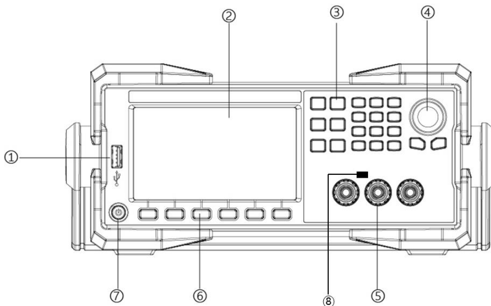
UDP69100/UDP69200/UDP69360 机型前面板
