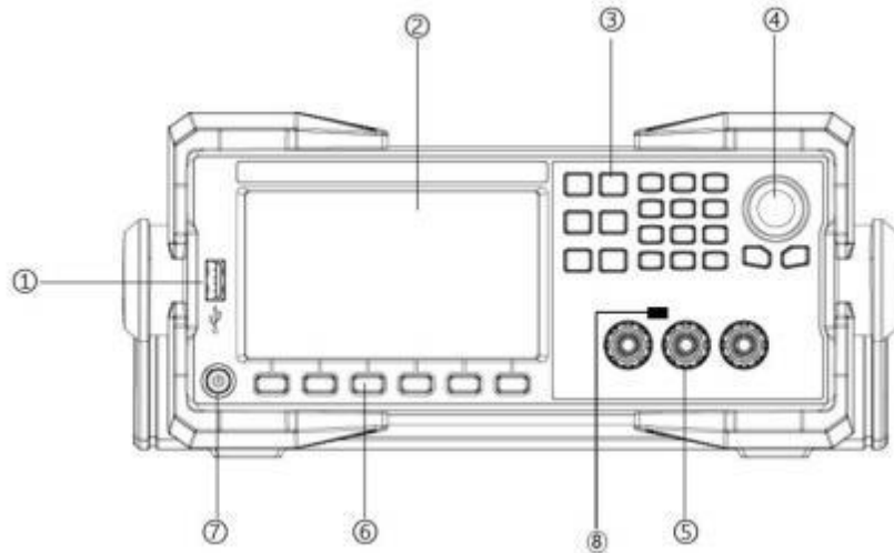
UDP6922B/UDP6932B/UDP6933B/UDP6942B/UDP6952B/UDP6953B 机型前面板
