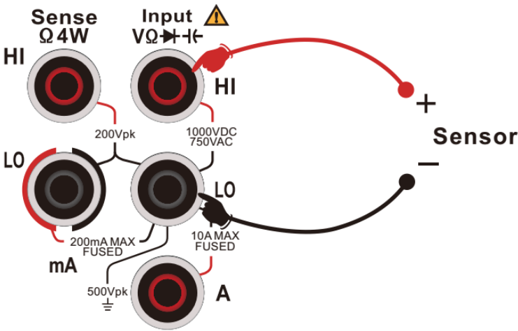
图 2 - 35温度测量接线示意图
