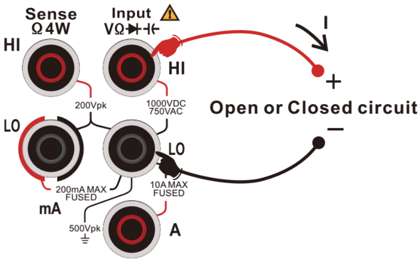
图 2 - 31 连通测量连接示意图
