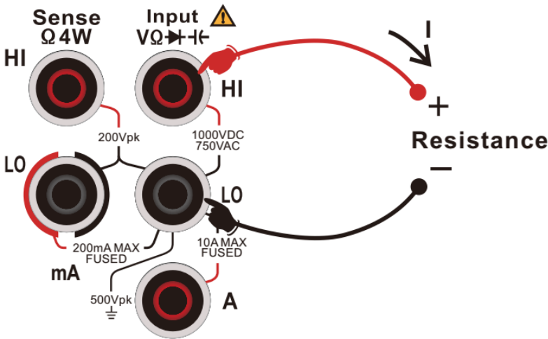
图 2 - 21 二线电阻测量连接示意图
