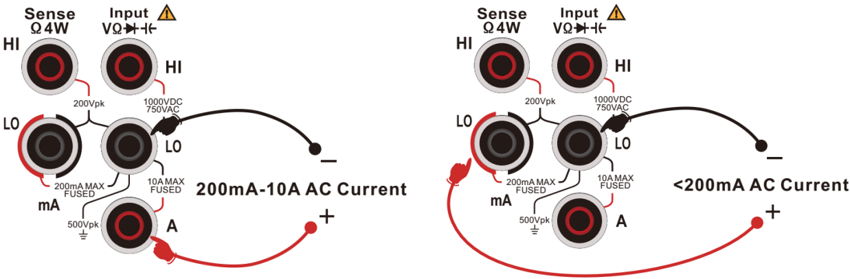
图 2 - 18交流电流测量连接示意图
