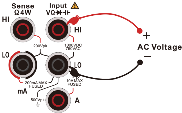
图 2 - 27信号频率测量连接示意图
