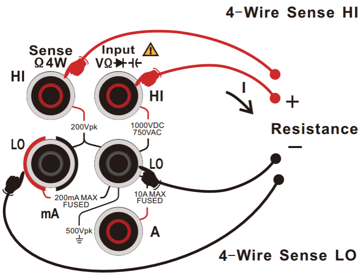
图 2 - 23四线电阻测量连接示意图
