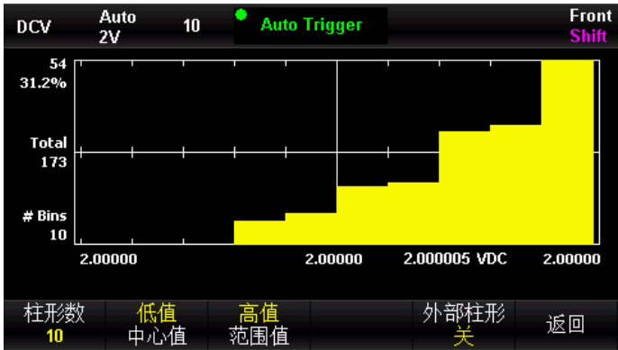
图 2 - 62直方图手动设置界面
