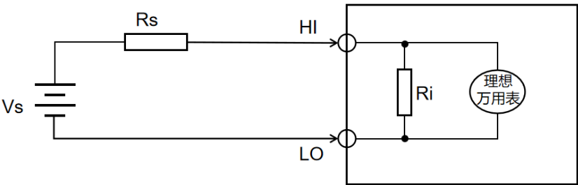
图 2 - 64 误差来源示意图
