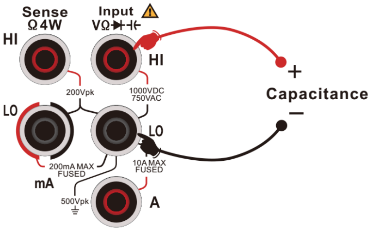
图 2 - 25电容测量连接示意图
