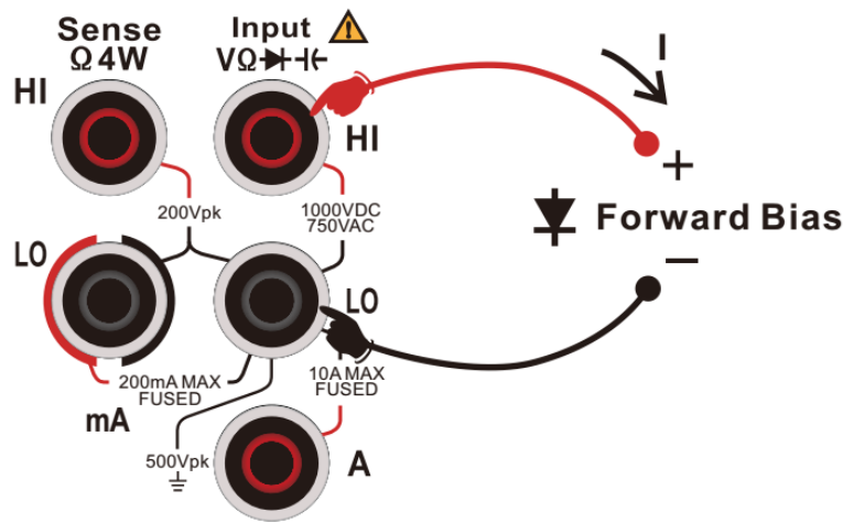
图 2 - 33 二极管测量连接示意图
