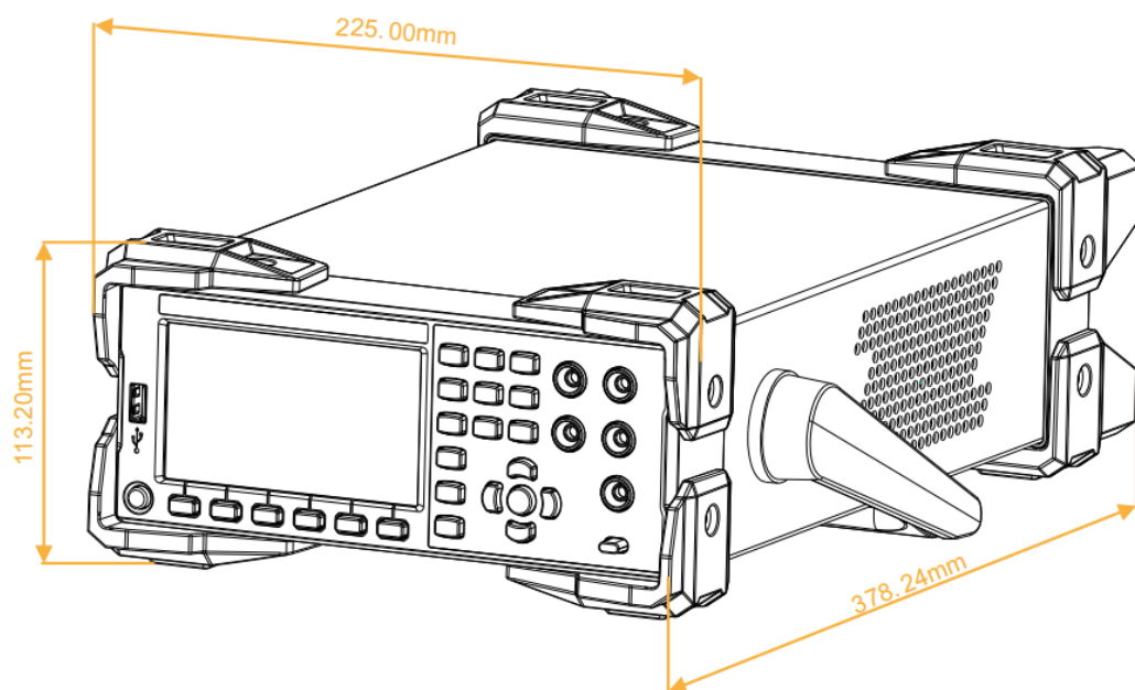
图 1 - 4 外观尺寸
