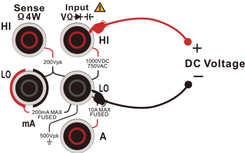
图 2 - 11 直流电压测量连接示意图
