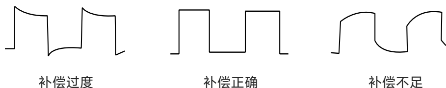
探头补偿校正
