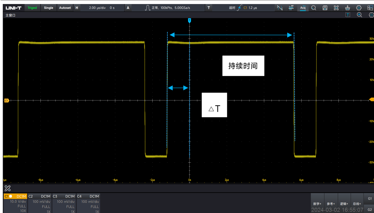
\Delta T > 持续时间触发
