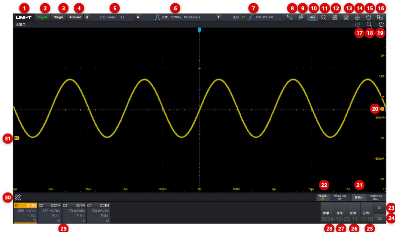
图 5 用户界面
