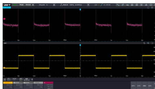
增强分辨率 3 位：噪声大约 3mV
