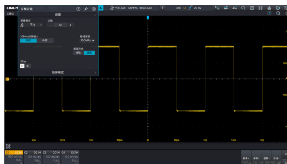
采用 32 次平均的波形
