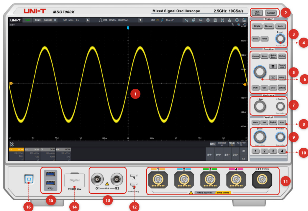
示波器前面板
